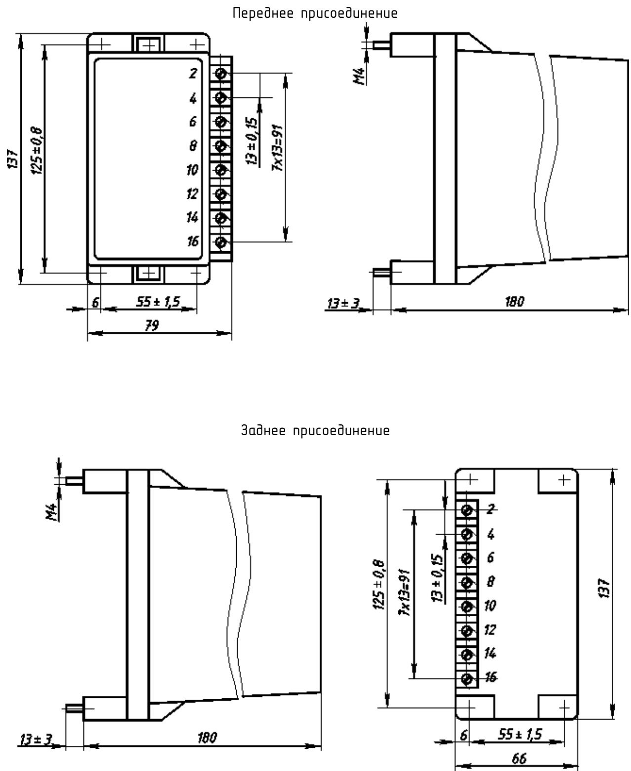
Рисунок В.1 – Габаритные, установочные и присоединительные размеры реле ООО «РЕОН-ТЕХНО»
